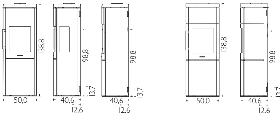
HWAM 4560m mit Specksteinverkleidung
