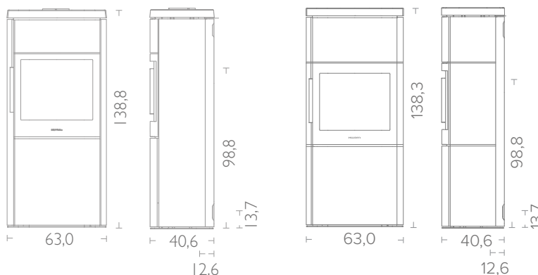
HWAM 4660m mit Tobacco Sandsteinverkleidung
