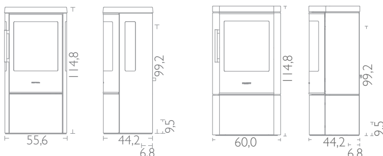
HWAM 3630c mit Seitenscheiben
